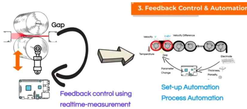
그림. 간극 측정/제어에 기반한 공정 자율화, 모니터링 및 이상진단 컨셉도
