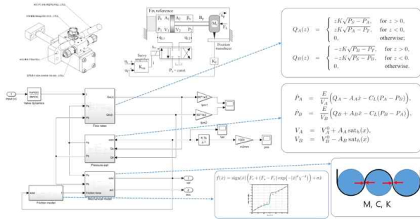
그림. 유압실린더 제어 동역학 모델 (볼프레스 제어용 동역학 모델로 확장 필요)
