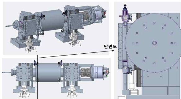
그림. On-machine 설치 가능한 간극 센서 설치(안)
